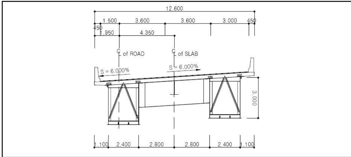
【그림 2.1.7】 해석단면
