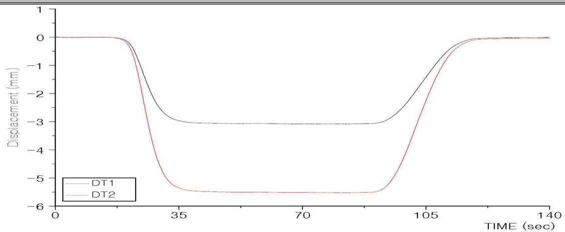
L.C3 처짐
