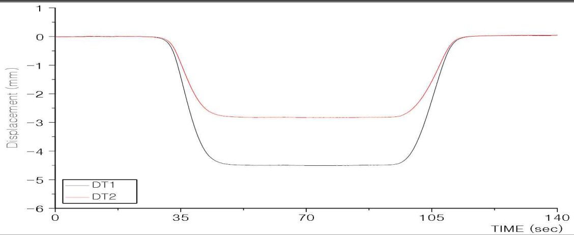
L.C2 처짐
