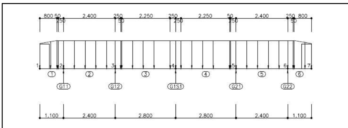
【그림 2.1.8】 바닥판 자중 횡방향 하중분배
