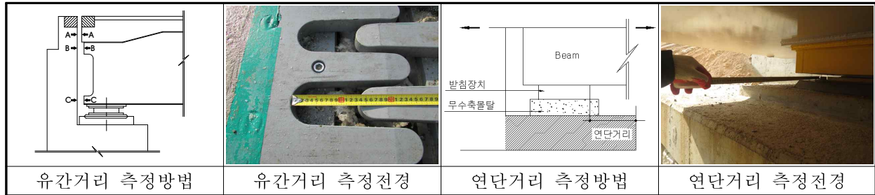
【그림 2.1.5】 부재별 기능상태 측정방법 및 전경
