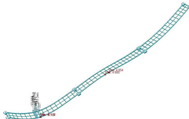
L.C3 하중재하 및 처짐
