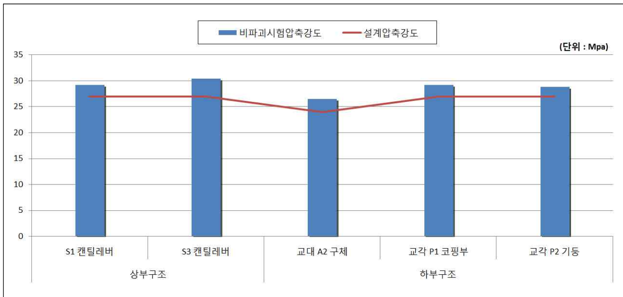
【그림 2.1.6】 콘크리트 강도시험 결과 그래프
