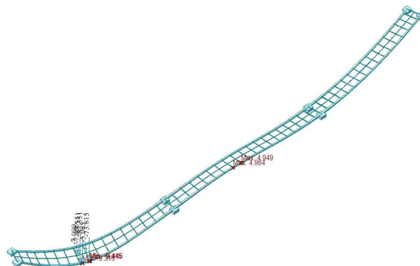
L.C3 하중재하 및 처짐
